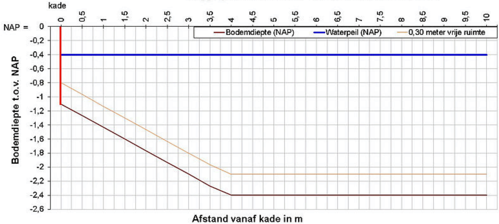
Leggerprofiel WEILG002 - t.h.v. Binnenkant 14 t/m 45
